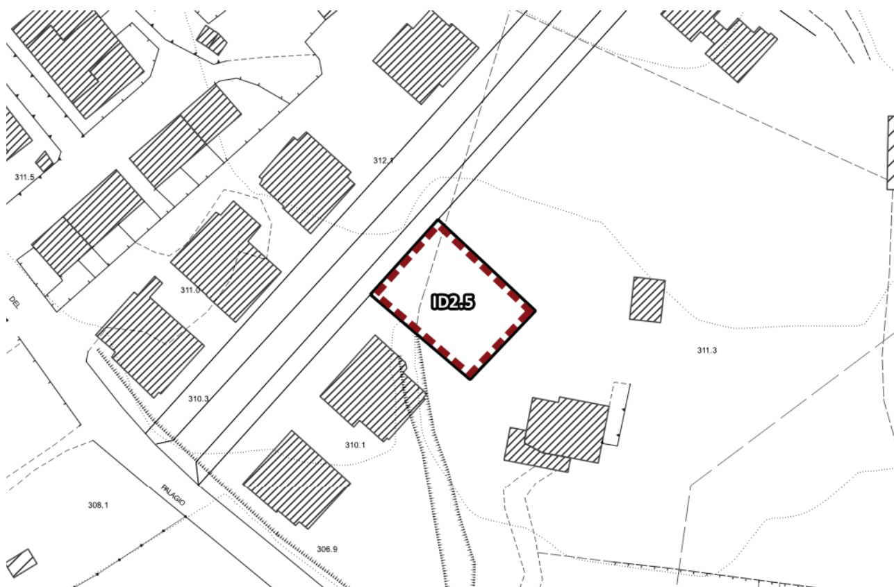
Individuazione vincoli sovraordinati – scala 1:1.000
